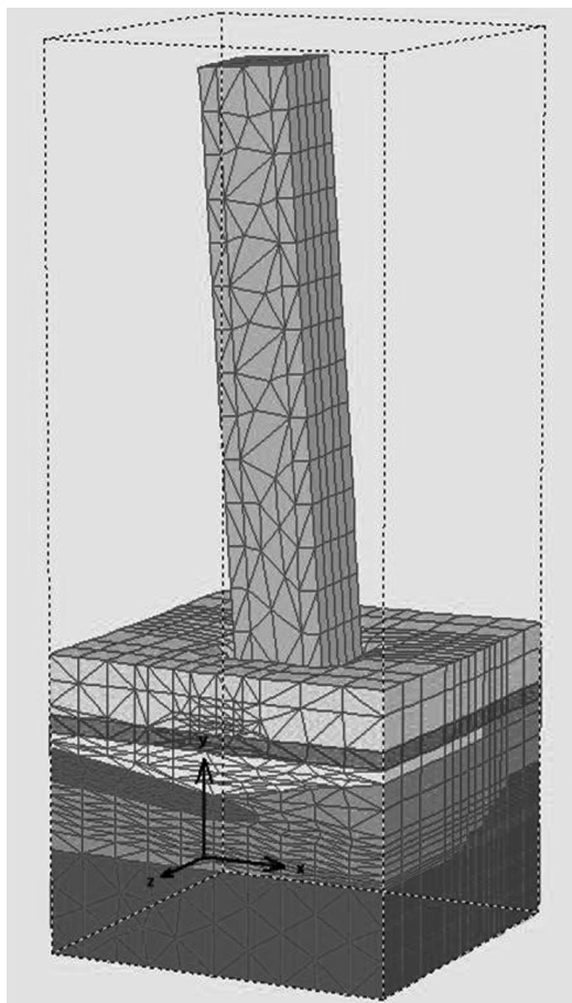
Fig. 5: Città di Castello tower mesh for the FEM analysis.
